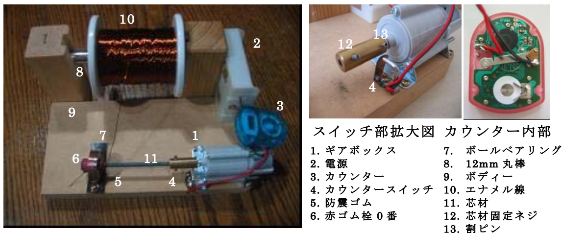
図1. コイルメーカー概観図
