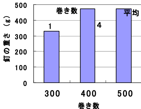
(a) 巻き数の影響
